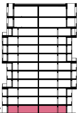
ŘEZ
